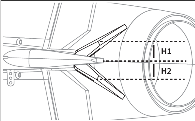
Seitenruder / Rudder
